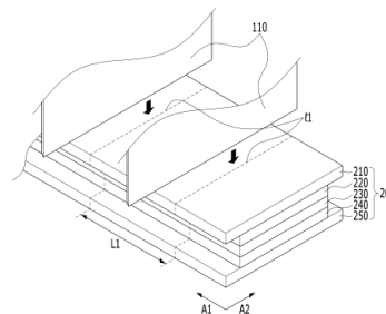
<점착필름 프레싱 방법 개요도>
